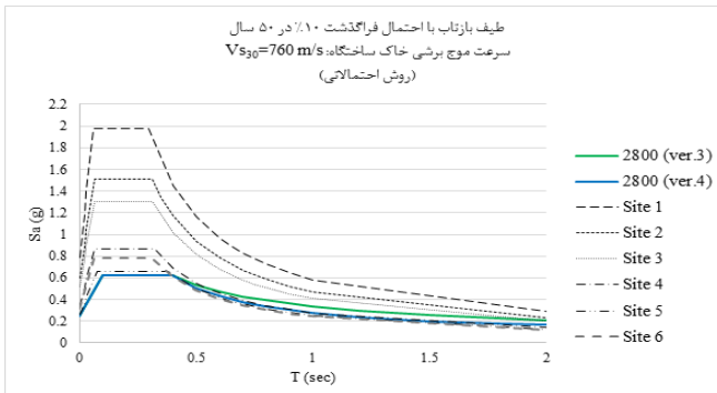
شکل ۷: مقایسه شتاب طیفی Sa(T) با استاندارد ۲۸۰۰ (ویرایش ۳ و ۴) به صورت A \times B(T) برای ۶ ساختمان که در آنها فقط اثرات گسل‌های اهواز و دزفول لحاظ شده است، بر روی خاک نوع ۱
