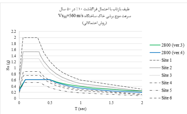
شکل ۸: مقایسه شتاب طیفی Sa(T) با استاندارد ۲۸۰۰ (ویرایش ۳ و ۴) به صورت A \times B(T) برای ۶ ساختمان که در آنها فقط اثرات گسل‌های اهواز و دزفول لحاظ شده است، بر روی خاک نوع ۲
