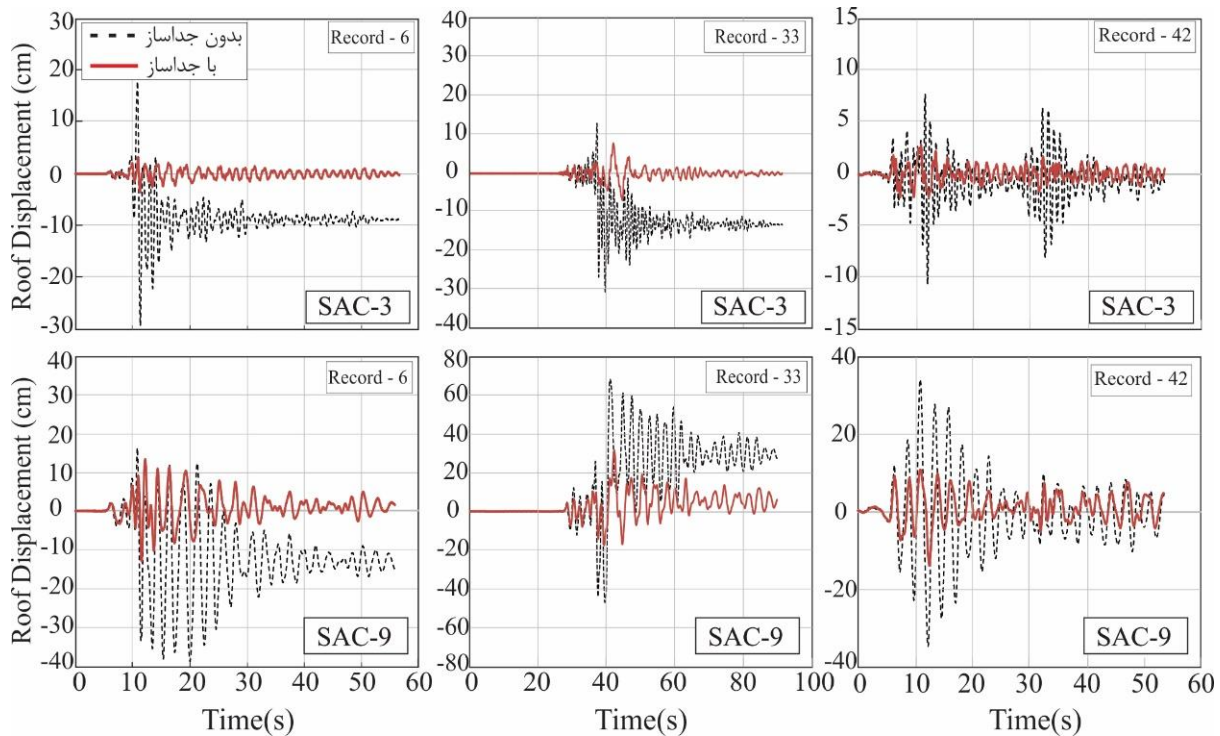
شکل ۱۵. نمودار تاریخچه زمانی جابه‌جایی بام سازه ۳ و ۹ طبقه سازه معیار SAC بدون جداساز و با جداساز
