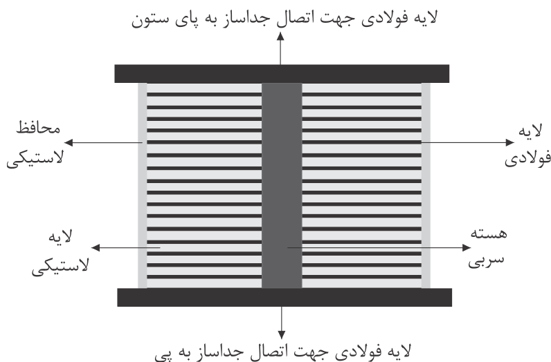
شکل ۳. شکل شماتیک جداساز سرب - لاستیکی
