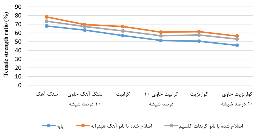
شکل ۱۴. نسبت مقاومت کششی غیرمستقیم (TSR) نمونه‌های ساخته شده با قیر ۶۰-۷۰ تحت سه دوره سیکل یخ - ذوب
