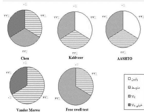
شکل (۱۷): تخمین تورم‌پذیری گمانه ۴ با استفاده از معیارهای آشتو، کالدویر، چن، واندرمر و تورم نسبی آزاد
