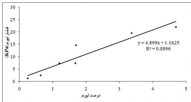
شکل (۲): رابطه بین درصد تورم و فشار تورم
