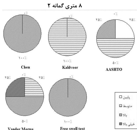
شکل (۷): تخمین تورم‌پذیری گمانه ۲ با استفاده از معیارهای آشتو، کالدویر، چن، واندرمر و تورم نسبی آزاد
