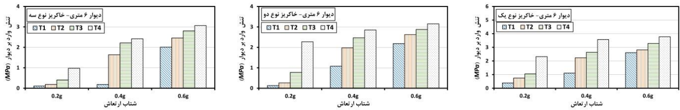
شکل ۱۲. تاثیر نوع خاکریز بر حداکثر تنش قائم وارد بر دیوار حائل ۶ متری
